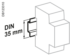
Montaggio su guida DIN 35 mm
