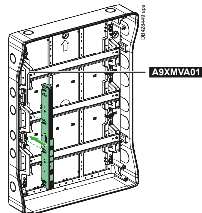
Armadio Mureva Enclosure montaggio verticale
