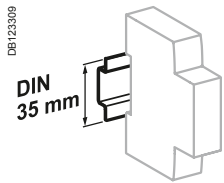
Aggancio su guida DIN da 35 mm
