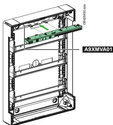
Armadio Pragma montaggio orizzontale
