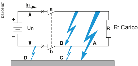
La figura rappresenta un'alimentazione in un sistema IT, con un secondo guasto (D) sulla polarità negativa.
