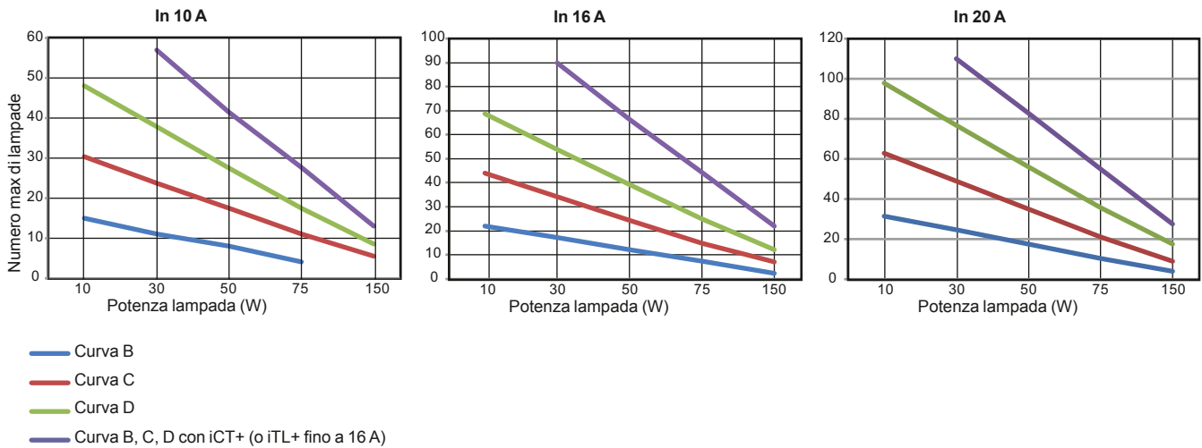
Numero max di lampade in base al calibro dell'interruttore e alla curva
